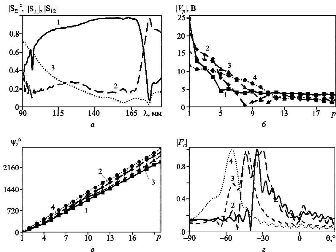
Рис. 6. Энергетические характеристики (а), амплитудные (б) и фазовые (в) распределения и диаграммы направленности (з) щелевой антенны, выполненной на фидере 2, l = 0.5L = 65 мм
