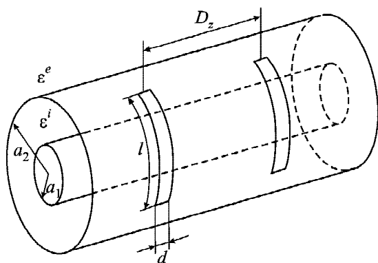
Рис. 1. Геометрия системы
