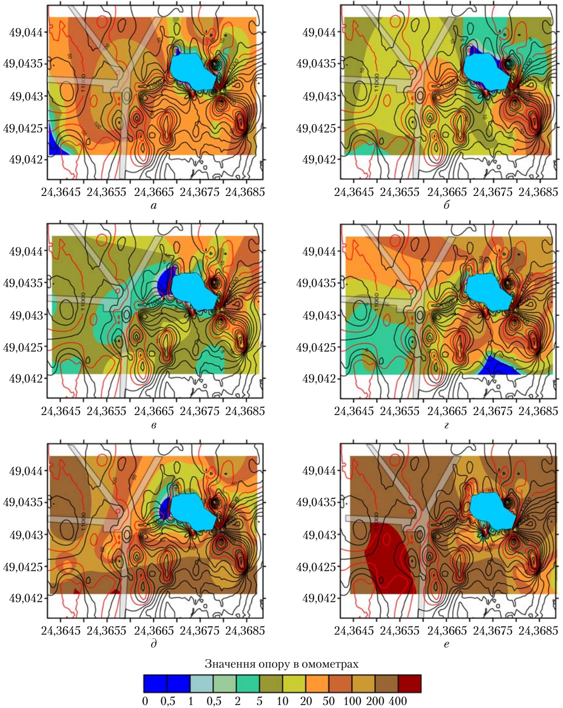
Рис. 5. Глибинні зрізи площинного розподілу питомого опору за даними ЗСБ та ізолінії інтенсивності ( N_v/c ) сигналів ПЕМПЗ на денній поверхні, ізолінії червоного кольору відповідають значенням, більшим за 10 000
