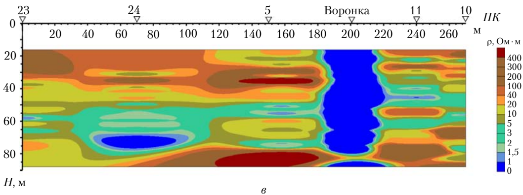
Рис. 4. Результати ЗСБ ділянки Північного карбінитового поля в районі карстового провалу (вул. Вітовського): a – розташування профілів I–I – VIII–VIII та підземних камер шатного поля, б – геоелектричний розріз вздовж профілю IV–IV, в – геоелектричний розріз вздовж профілю V–V, що пересікає провальну воронку
