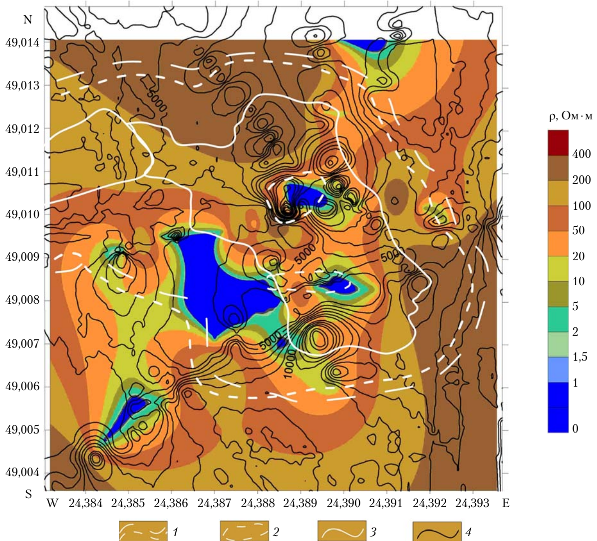
Рис. 8. Глибинний зріз площинного розподілу питомого опору на глибині 45 м у комплексі з розподілом ПІЕМПЗ та інженерно-геологічними даними: 1 – границі мульки за інженерно-геологічними визначеннями, 2 – області найбільшого просідання, 3 – границі шахтного поля, 4 – ізолінії розподілу вертикальної компоненти ПІЕМПЗ
