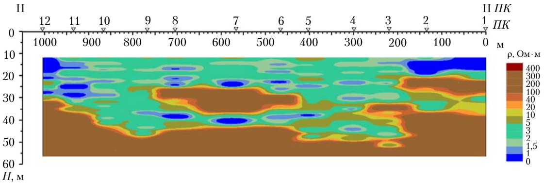
Рис. 7. Мережа профілів ЗСБ (I–I – IV–IV) та ШЕМПЗ на Хотінському сільвінітовому полі. Нижче – геоелектричний розріз вздовж поперечного профілю II–II
