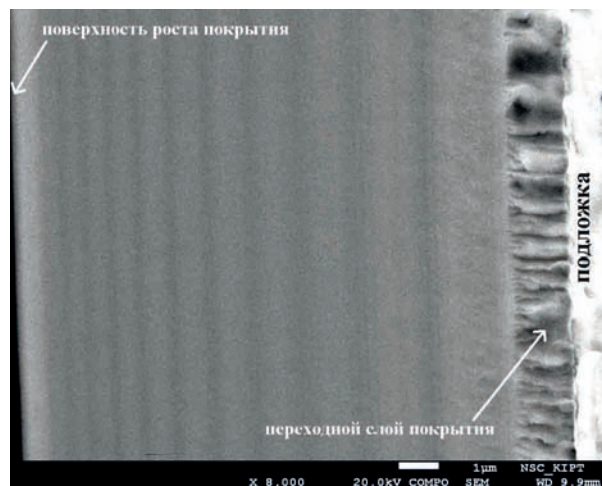
Рис. 5. Слоистое покрытие пиролитического хрома, полученного при T_{oc} = 500\text{ }^{\circ}\text{C} на медной подложке; средняя скорость осаждения 4,5\text{--}6\text{ мкм/мин} ; отношение S/V = 6\text{ см}^{-1}
