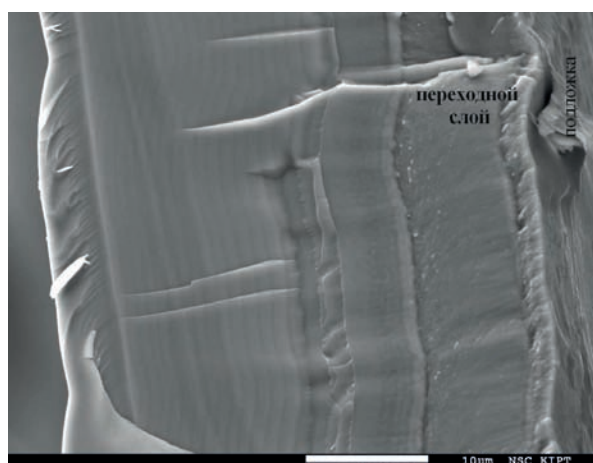
Рис. 6. Слоистое покрытие пирохромического хрома, полученного при T_{oc} = 500 °С на алюминиевой подложке; средняя скорость осаждения 1–1,2 мкм/мин; отношение S/V = 0,065 см -1
