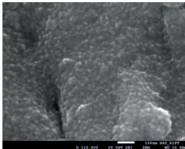
Рис. 8. Поверхность скола слоисто-столбчатого пиrolитического карбидохромового покрытия толщиной 18 мкм, полученного при температуре осаждения 500 °С, отношение S/V = 0,08\text{см}^{-1} , средняя скорость осаждения — 0,9 мкм/мин, \times 110,000
