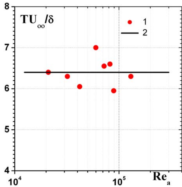
Рис. 9. Период генерации наибольших когерентных вихревых структур пограничного слоя на цилиндре
