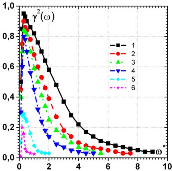
Рис. 2. Залежності функцій когерентності от частоти для різних відстаней між датчиками пульсацій тиску
