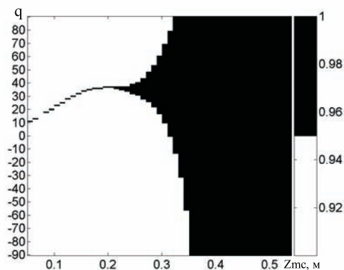
Рис. 23. Рельеф AP-оценки угловой СПМ сигнала сосредоточенного источника в коаксиально-слоистой цилиндрической трубе при скоростях звука в слоях C_1 = C_3 = 23 м/с и C_2 = 45 м/с
