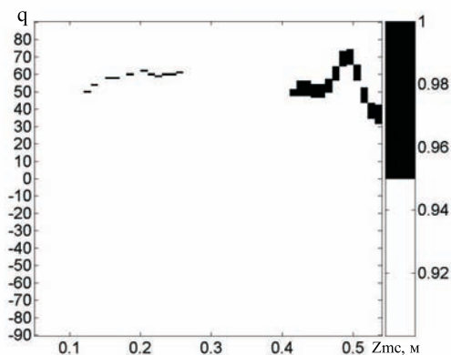
Рис. 10. Рельеф угловой СПМ сигнала сосредоточенного источника для алгоритма АР-оценивания в однородной цилиндрической трубе при скорости звука C_o = 45 м/с
