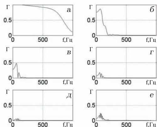
Рис. 2. Частотные зависимости функций когерентности сигнала протяженного источника в однородной цилиндрической трубе со скоростью звука C_0 = 23 м/с в полосе (382...632) Гц при использовании двухэлементных антенн с разными дистанциями между приемниками: а - \Delta z = 0.01 м, б - \Delta z = 0.1 м, в - \Delta z = 0.2 м, г - \Delta z = 0.3 м, д - \Delta z = 0.4 м, е - \Delta z = 0.5 м
