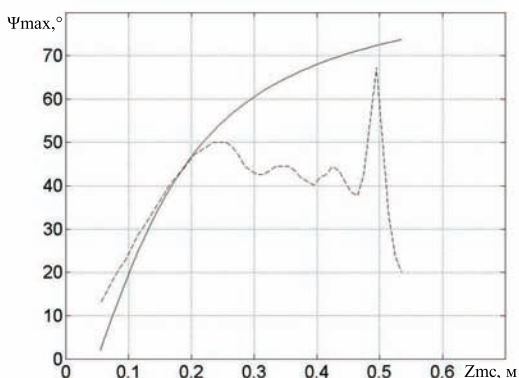
Рис. 11. Сравнение траектории АР-оценок направлений максимумов \Psi_{\max} угловых спектров сигнала сосредоточенного источника (штриховая) с траекторией геометрических направлений из центра базы антенны на источник (сплошная) для однородной трубы со скоростью звука в стенке C_o = 45 м/с
