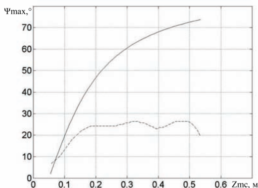
Рис. 24. Сравнение траектории AP-оценок направлений максимумов угловых спектров сигнала сосредоточенного источника (штриховая) с траекторией геометрических направлений на источник из центра базы антенны (сплошная) для коаксиально-слоистой цилиндрической трубы при скоростях звука в слоях C_1 = C_3 = 23 м/с и C_2 = 45 м/с
