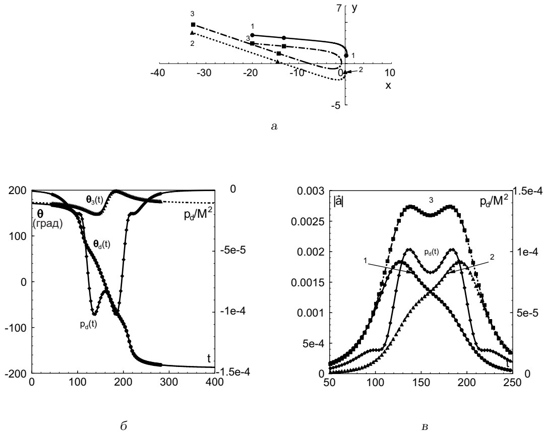
Рис. 8. Поведение системы при b=2.95 :
