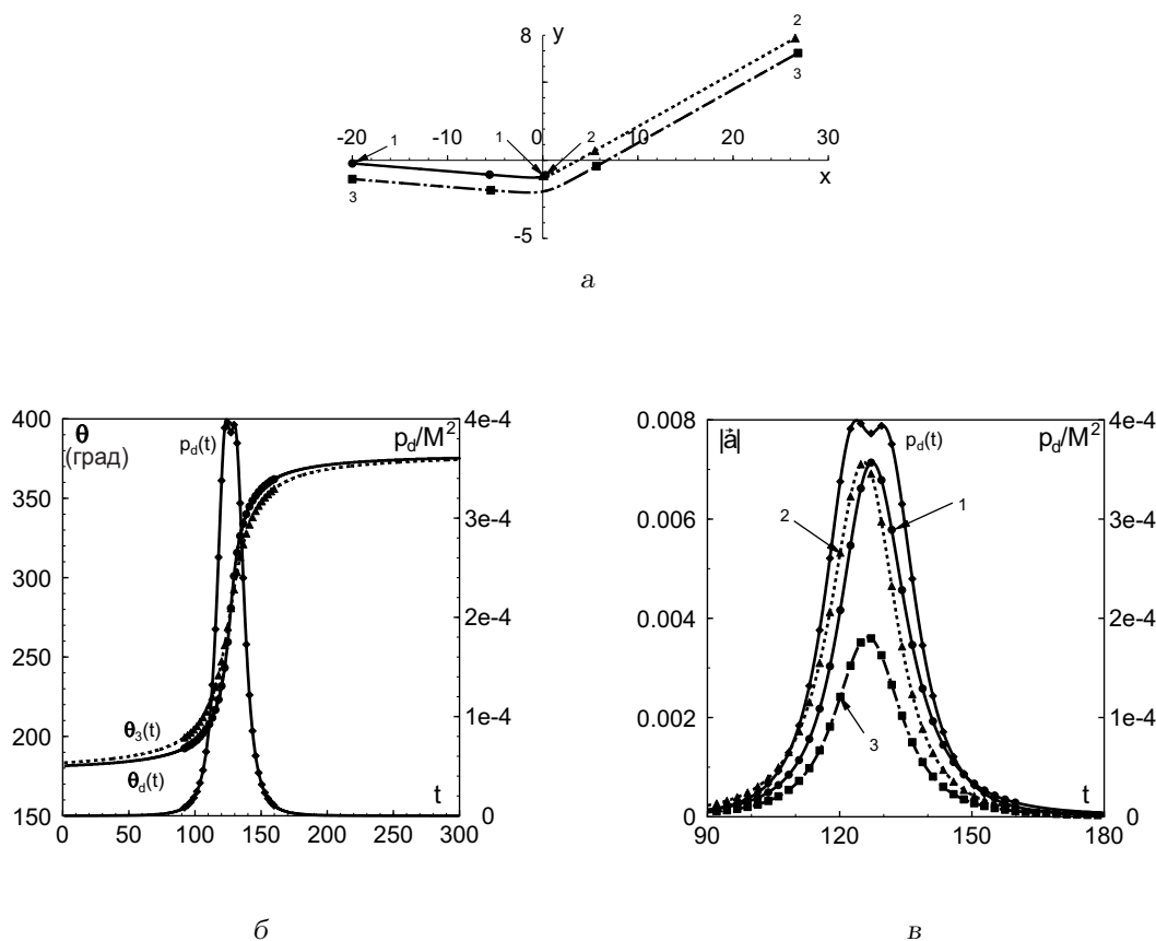
Рис. 3. Поведение системы при b = -0.7 :
