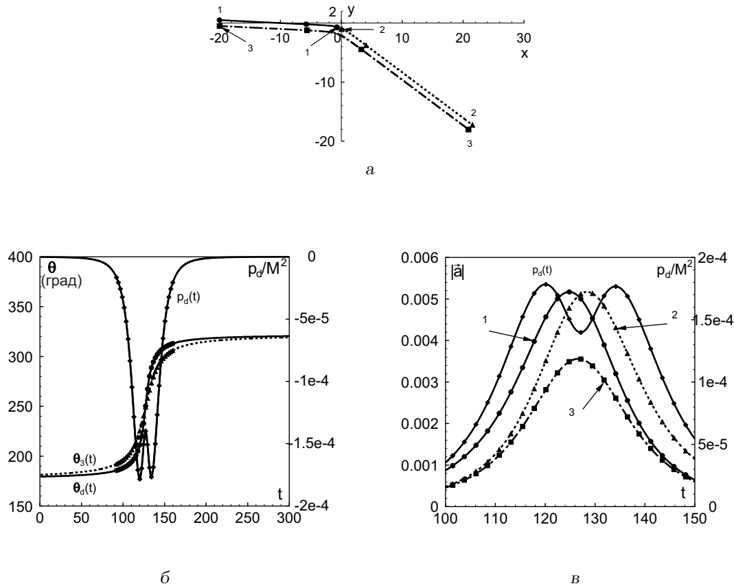
Рис. 4. Поведение системы при b=0 :
