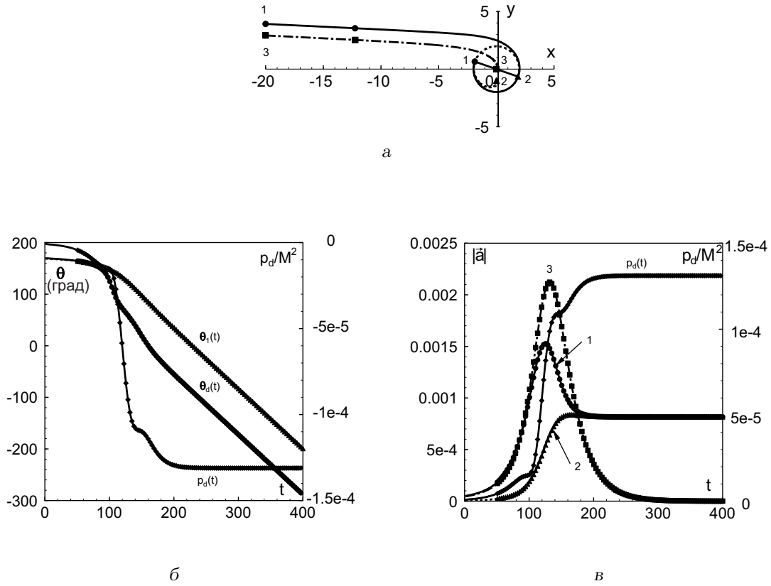
Рис. 14. Поведение системы при b=3.41 \dots :
