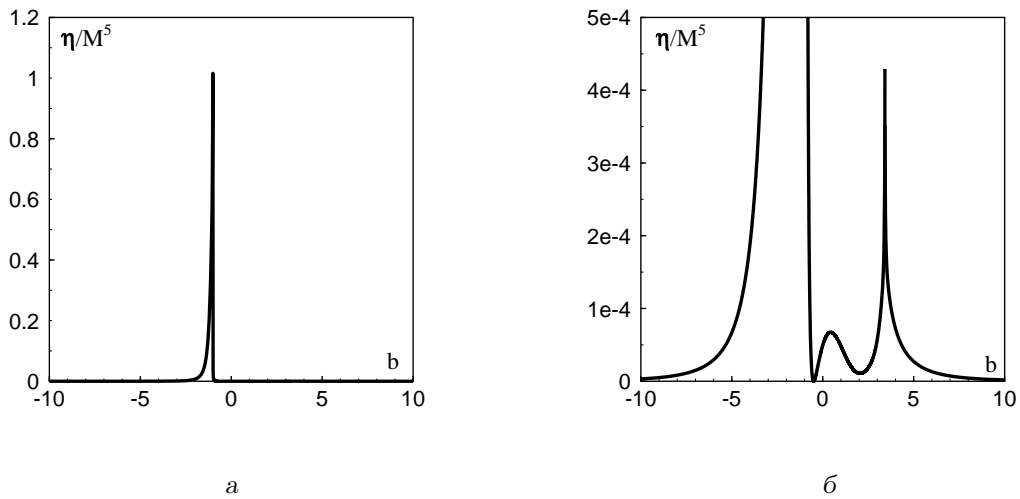
Рис. 15. Зависимость эффективности излучения вихрей от параметра b :
