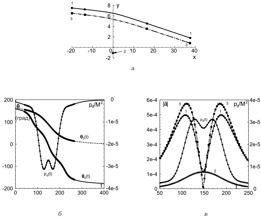
Рис. 10. Поведение системы при b=7.0 :
