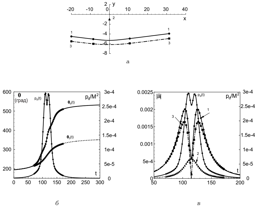
Рис. 2. Поведение системы при b = -5 :
