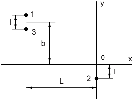
Рис. 1. Начальная геометрия модельного течения: 1,3 – падающая вихревая пара; 2 – одиночный вихрь
