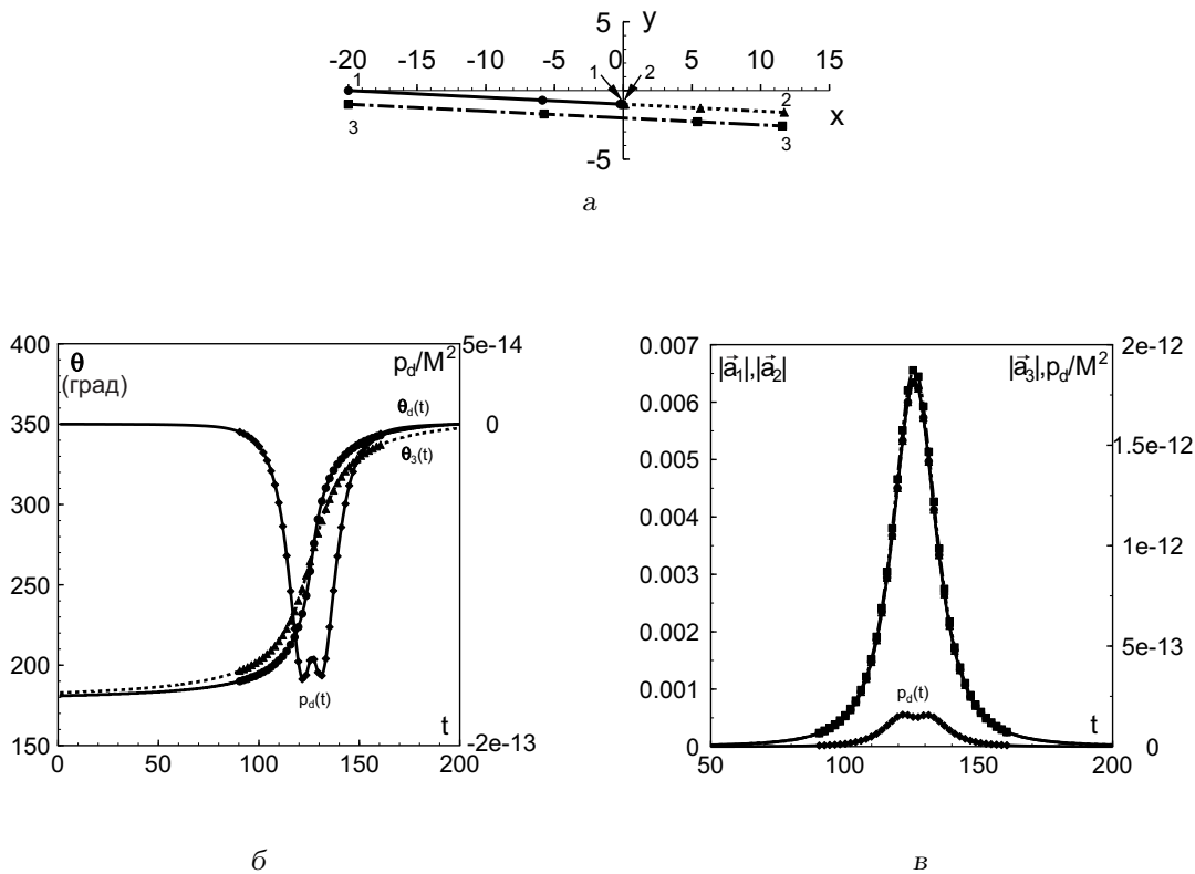
Рис. 13. Поведение системы при b = -0.5 :
