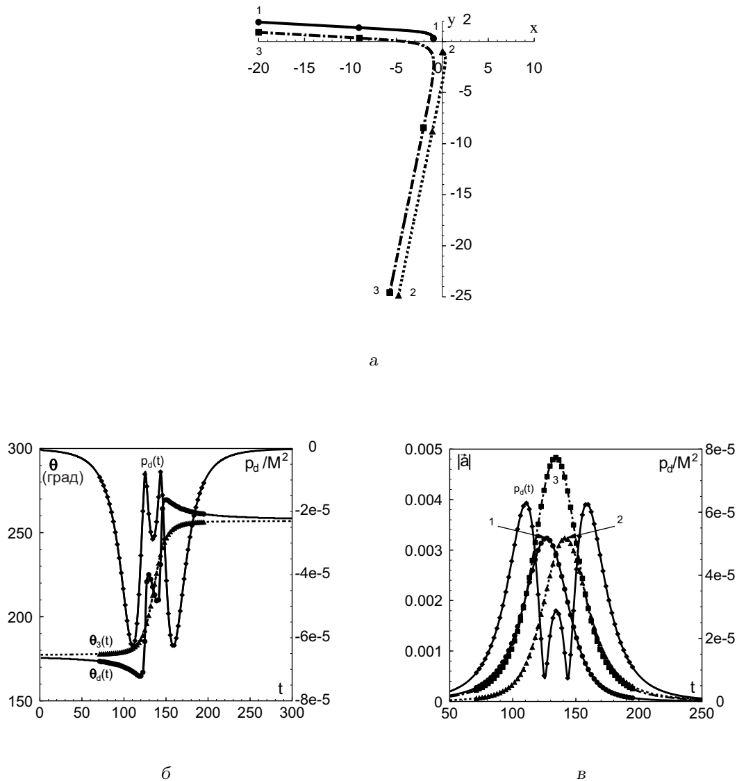
Рис. 5. Поведение системы при b=1.4 :
