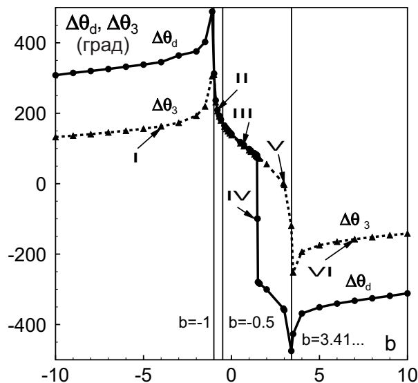
Рис. 11. Зависимости полного поворота диаграммы направленности \Delta\theta_d(b) (сплошная) и вихревой системы \Delta\theta_3(b) (штриховая) от параметра b
