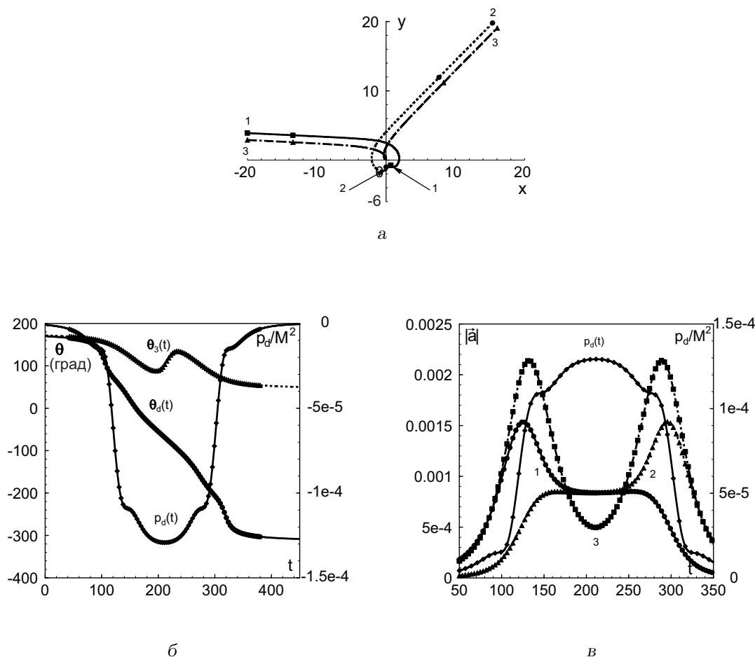
Рис. 9. Поведение системы при b = 3.4 :
