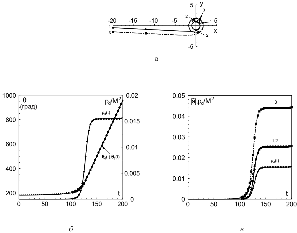
Рис. 12. Поведение системы при b = -1 :
