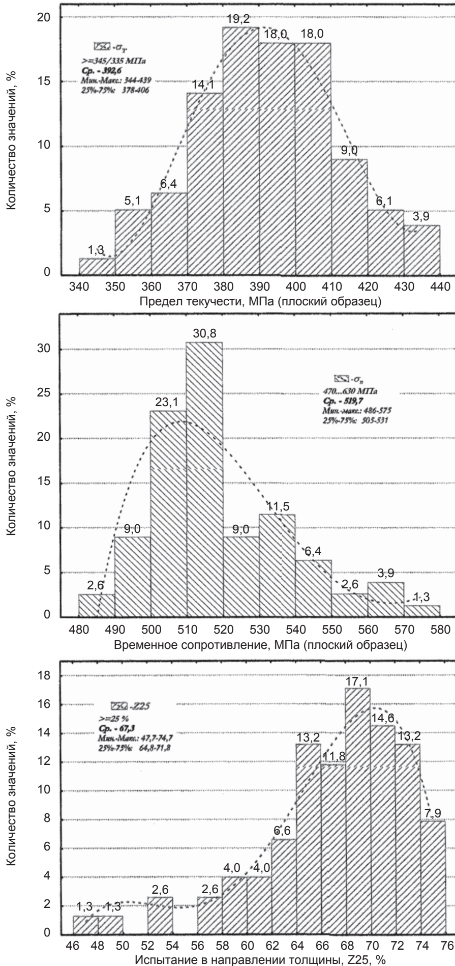
Рис. 3. Уровень механических свойств плит толщиной более 32 мм, количество значений – 78 шт. S355...N (+Z25), EN 10025-2:2004, шифр 9.324. ЛПЦ-3000
