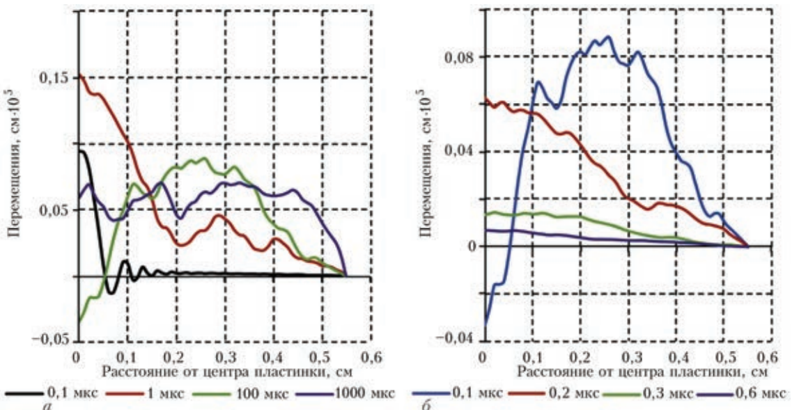
Рис. 3. Колебания пластинки с закрепленными краями в зависимости от времени (а) и толщины (б) (графики на этом рисунке представлены для 0,0001 с после начала действия источника)
