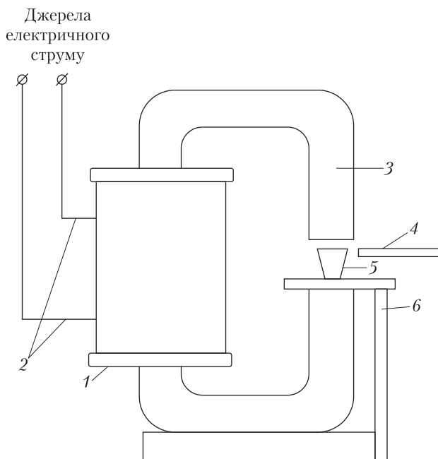
Рис. 2. Схематичне зображення конструкції комбінованого пристрою, що містить джерела магнітного поля 1,3 та кровопливу (ДКВ) 4: 1 – котушка; 2 – електричні вводи котушки; 3 – феромагнітне осердя; 4 – джерело кровопливу; 5 – кювета з піддослідним об'єктом; 6 – висувний столик для фіксації піддослідних об'єктів
