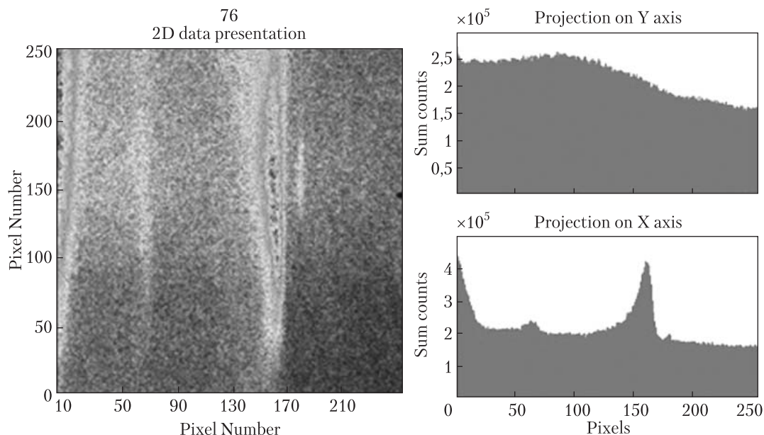
Рис. 3. Зліва — розподіл інтенсивності рентгенівських квантів, розсіяних на металевому зразку, виміряний кремнієвим детектором TimePix в установці швидкісного рентгенографування. Справа — проєкції цього двовимірного розподілу на осі Y та X
