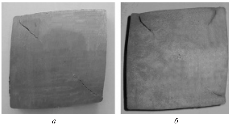
Рис. 5. Характерное расположение диагональных трещин на поперечных темплетях (квадрат 125 мм) сортовой заготовки: а — 18 мм, б — 16 мм (ромбичность)
