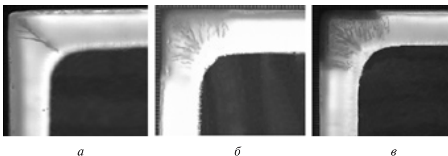
Рис. 3. Характерный вид твердой корочки заготовки после затвердевания в кристаллизаторе: a — без теплоизолятора; б и в — с теплоизоляторами толщиной 1 и 2 мм, установленными в углу кристаллизатора
