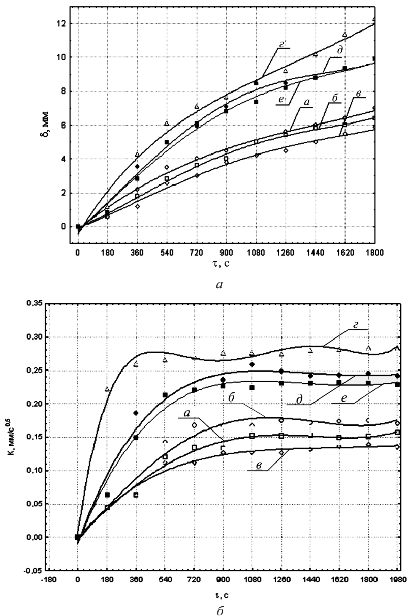
Рис. 2. Динамика продвижения фронта затвердевания (а) и изменения коэффициента затвердевания (б) в зависимости от режима охлаждения граней модели: а, а' – интенсивность охлаждения 0,818 л/мин; б, б' – интенсивность охлаждения 0,409 л/мин; в, в' – интенсивность охлаждения 0,080 л/мин
