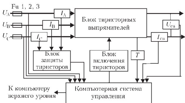
Рис. 1. Структурная схема преобразователя
