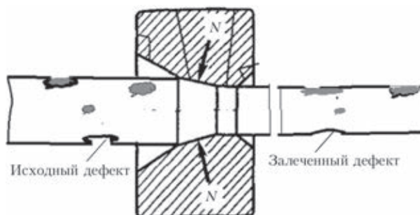
Рис. 8. Схема формирования дефектов на поверхности проволоки при волочении
