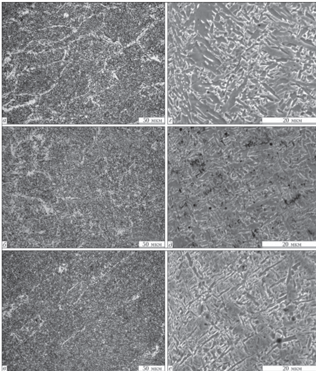
Рис. 5. Микроструктура металла исследованных швов: а, з — шов \text{TiO}_2 ; б, д — шов \text{TiC} ; в, е — шов \text{TiN}
