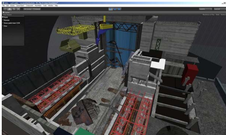
Рис. 4. Вигляд ЦЗ після демонтажу перекриття приміщень південних та північних барабан-сепараторів.
