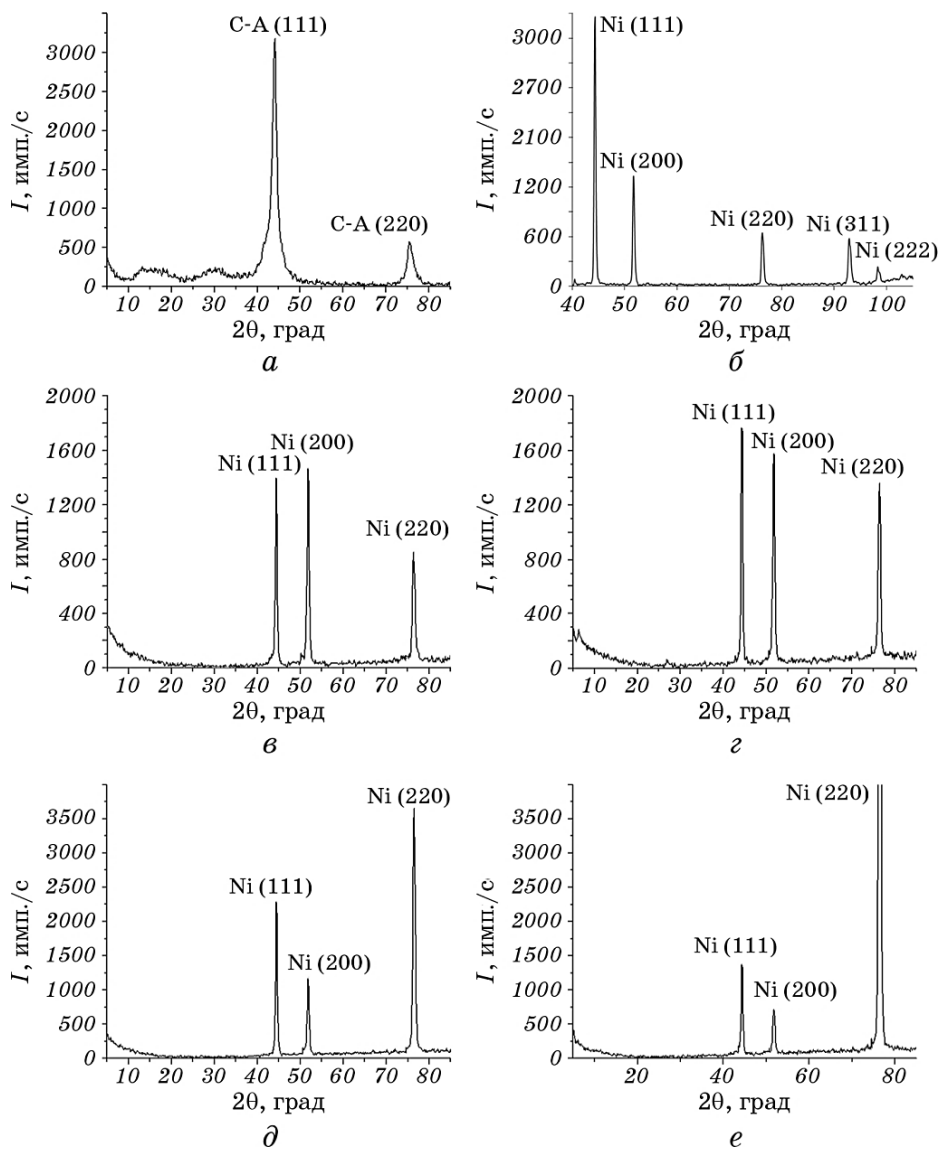
Рис. 1. Дифрактограммы УДА (а), Ni (эталон) (б), а также Ni + УДА, осаждённых с помощью как постоянного ( j = 100 \text{ А/м}^2 ) (в), так и импульсного тока ( f = 50 \text{ Гц} , j_{\text{cp}} = 100 \text{ А/м}^2 ): Ni + УДА ( Q = 2 ) (г), Ni + УДА ( Q = 25 ) (д), Ni + УДА ( Q = 50 ) (е).
