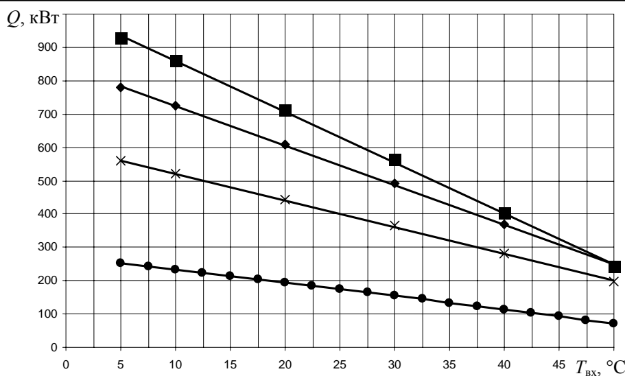
Рис. 4. Зависимость отбираемой тепловой мощности от температуры теплоносителя на входе при времени непрерывной эксплуатации 180 суток и расходе:
