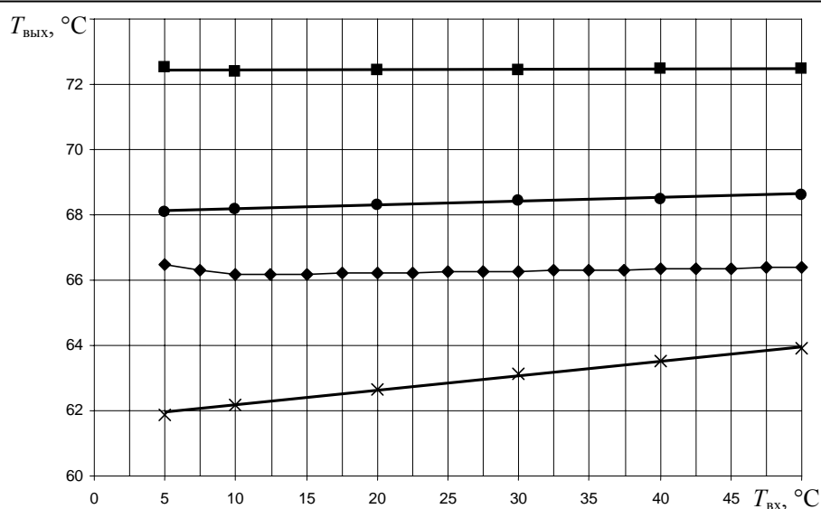
Рис. 3. Зависимость температуры теплоносителя на выходе от температуры на входе при времени непрерывной эксплуатации 180 суток и расходе:
