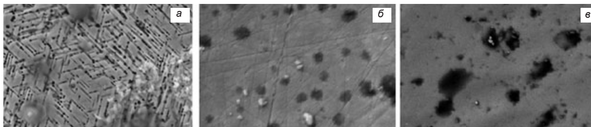
Рис. 1. Наноструктуры на поверхности полупроводников: a — InP, j = 80 мА/см 2 , t = 10 мин; б — GaAs, j = 60 мА/см 2 , t = 15 мин; в — GaP, j = 100 мА/см 2 , t = 5 мин
