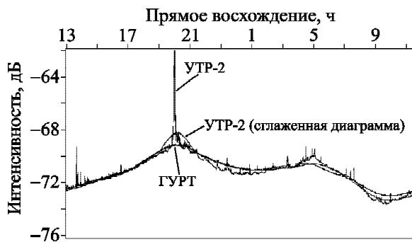
Рис. 17. Суточная зависимость интенсивности радиоизлучения фона Галактики в направлении точки кульминации радиоисточника 3С 405, полученная с помощью западного плеча УТР-2 и субрешетки ГУРТ
