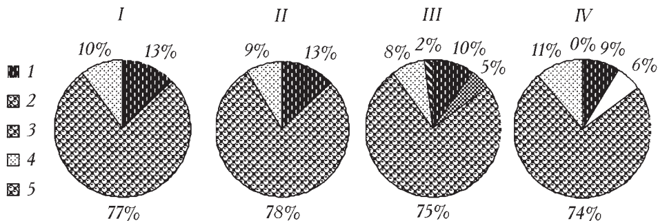
4. Співвідношення видів — індикаторів солоності води кар'єрів м. Житомира: 1 — олігогалоби; 2 — галофоби; 3 — індіференти; 4 — галофіли; 5 — мезогалоби.
