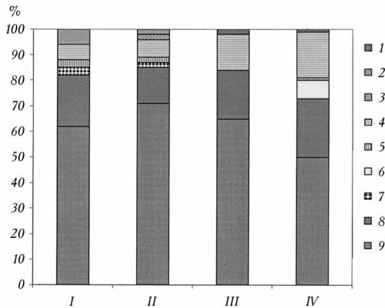
3. Розподіл водоростей кар'єрів м. Житомира за біотопічною приуроченістю: 1 — бентосно-планктонні; 2 — планктонно-епіфітні; 3 — планктонно-літоральні; 4 — бентосні; 5 — епіфітно-планктонні; 6 — види обростань; 7 — планктонно-бентосні; 8 — літоральні; 9 — планктонні.
