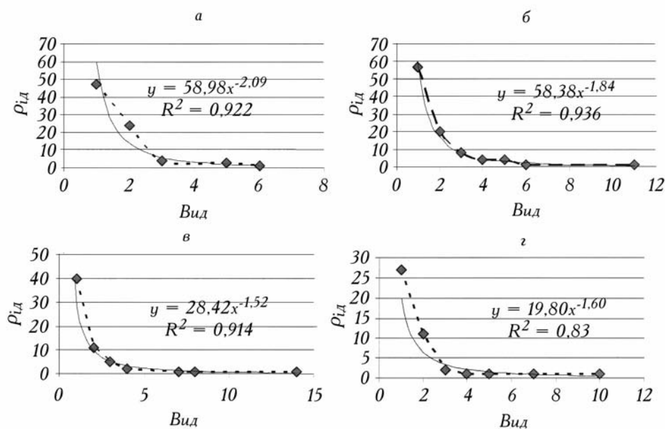
2. Залежність Віллса для альгофлор водойм антропогенного походження м. Житомира: а — Богунський кар'єр; б — кар'єр Сонячний; в — Слобідський кар'єр; г — Селецький кар'єр.
