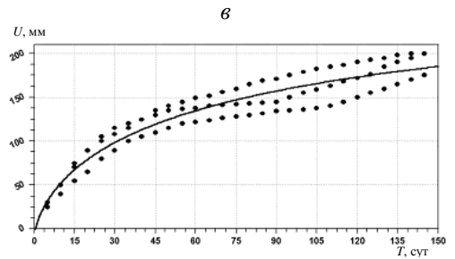
Рис. 4. Зависимость смещений контура выработки во времени для пород: а – кровли; б – почвы; в – боковых пород
