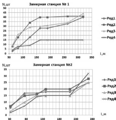
Рис. 6. Зависимость количества поломанной затяжки по периметру выработки от времени проведения выработки
