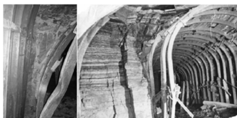
Рис. 2. Расслоение пород приконтурного массива
