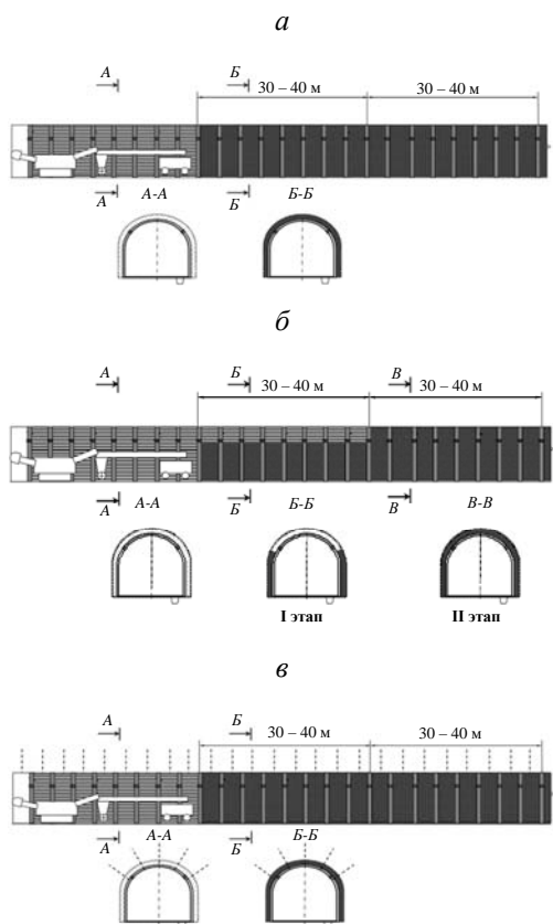
Рис. 9. Технологические схемы возведения крепи с тампонажем закрепного пространства: а – за один прием; б – в два этапа; в – с установкой анкеров
