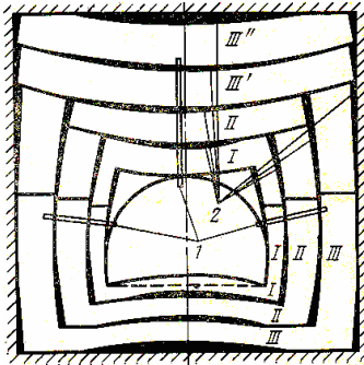
Рис. 3. Схема деформирования (разрушения) пород приконтурного слоя и образование зон разрушения: I, II, III – зоны разрушения вмещающего массива; 1 – шпурсы для тампонажа разрушенного массива; 2 – пустоты
