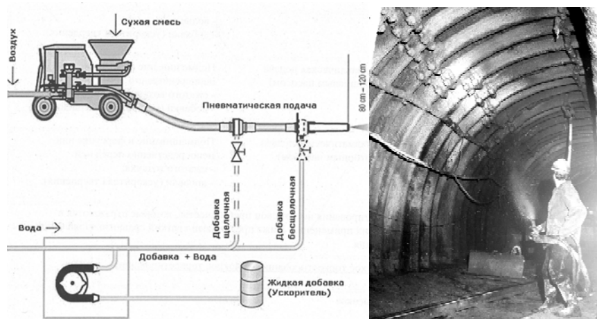
Рис. 8. Пневматическая подача смеси при сухом торкретировании
