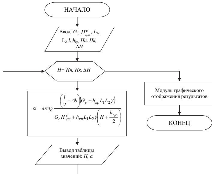
Рис. 2. Блок-схема алгоритма
