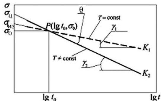
Рис. 5. Схематическое представление результатов термоциклических и изотермических испытаний тугоплавких сплавов на длительную прочность
