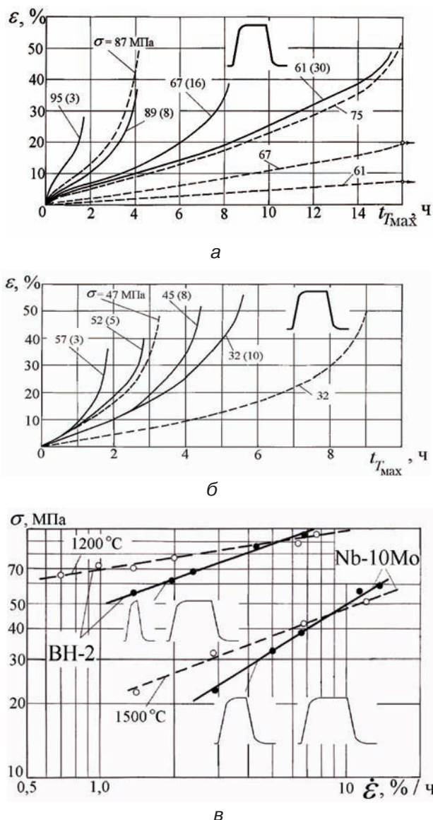
Рис. 3. Кривые ползучести (а, б) и скорость ползучести (в) сплавов на основе ниобия: а - ВН-2, T_{\max} = 1200 °С; б - Nb-10Mo, T_{\max} = 1500 °С; сплошные линии - термоциклирование, штриховые - изотермические испытания; в скобках указано число температурных циклов до разрушения образца
