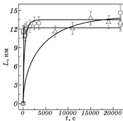
Рис. 3. Зависимость размеров нанокристаллов алюминия от времени для различных температур отжига: \triangle — 460 К, \circ — 501 К, \square — 536 К; сплошные линии — результат расчета по уравнению (4).
