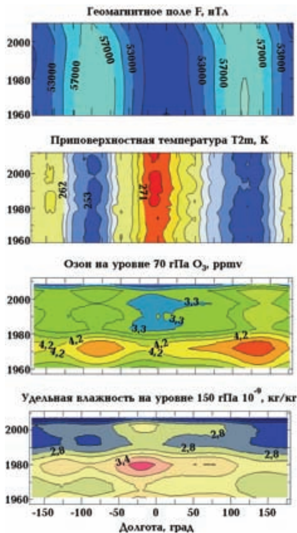
Рис. 1. Пространственно-временное распределение усредненных значений F, T2m, O 3 , SpH в диапазоне широт 40–70° с. ш. за период 1957–2011 гг.
