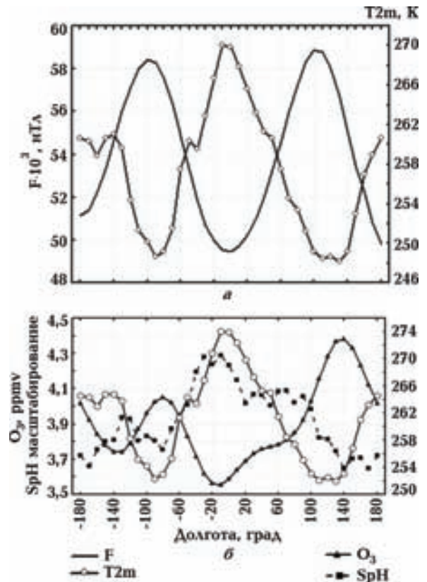
Рис. 2. Интегральные характеристики модуля полного вектора геомагнитного поля F и приземной температуры воздуха T_{2m} (а), приземной температуры воздуха T_{2m} , озона O_3 на уровне 70 гПа, удельной влажности SpH на уровне 150 гПа (б). Осреднение выполнено в широтном поясе 40—70° с. ш. за период 1957—2011 гг.
