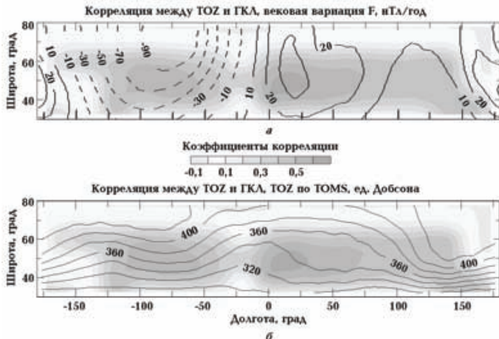
Рис. 6. Пространственно-временное распределение статистически значимых коэффициентов корреляции между ТОЗ (по TOMS) и ГКЛ (по Climax) за период 1980—2010 гг. Контурами приведены 30-летние средние значения вековой вариации геомагнитного поля, нТл (а) и озона, ед. Добсона (б).
