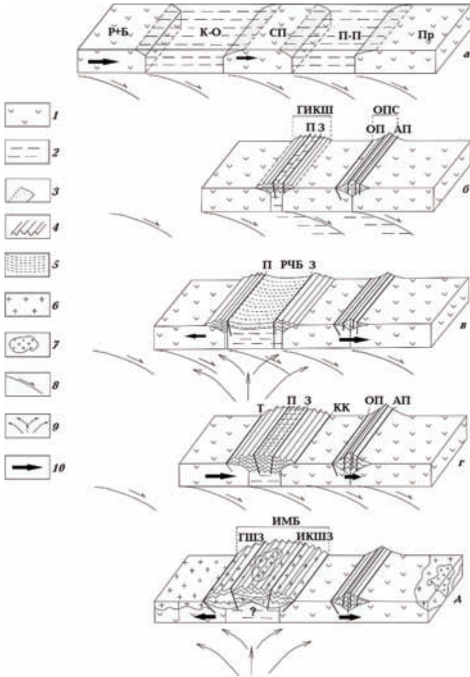
Рис. 5. Упрощенная немасштабная схема предполагаемого палеогеодинамического процесса в центральной и восточной части УЩ, по [Гинтов, 2014]: 1 — континентальные микроплиты, состоящие из архейских мегаблоков (Р + Б — Росинского и Бугского, СП — Среднеприднепровского, Пр — Приазовского); 2 — океанские (субокеанские) микроплиты (К-О — Криворожско-Одесская, П-П — Приднепровско-Приазовская); 3 — терригенно-вулканогенно-карбонатные толщи, откладываемые на континентальных окраинах (геоклиналях); 4 — складчатость в породах коллизионных швов; 5 — вулканогенно-осадочные образования Рощаховско-Чечелевского бассейна; 6, 7 — протерозойская гранитизация архейских мегаблоков (6 — 2,0—2,1 млрд лет назад, 7 — 1,75—1,8 млрд лет назад); 8, 9 — направление движения мантийного вещества (8 — в восточной ветви конвективной ячейки или мантийного плюма регионального масштаба, 9 — в пульсирующем мантийном плюме местного масштаба); 10 — направление перемещения континентальных плит (длина стрелки отражает условную относительную скорость перемещения плиты). Буквенные обозначения: ГИКШ — Голованевско-Ингулецко-Криворожский коллизионный шов, ОПС — Орехово-Павлоградская сутура, РЧБ — Рощаховско-Чечелевский бассейн, ИМБ — Ингульский мегаблок, ГШЗ — Голованевская шовная зона, ИКШЗ — Ингулецко-Криворожская шовная зона; зоны разломов: П — Первомайская, З — Западно-Ингулецкая, ОП — Орехово-Павлоградская, АП — Азовско-Павловская, Т — Тальновская, КК — Криворожско-Кременчугская.
