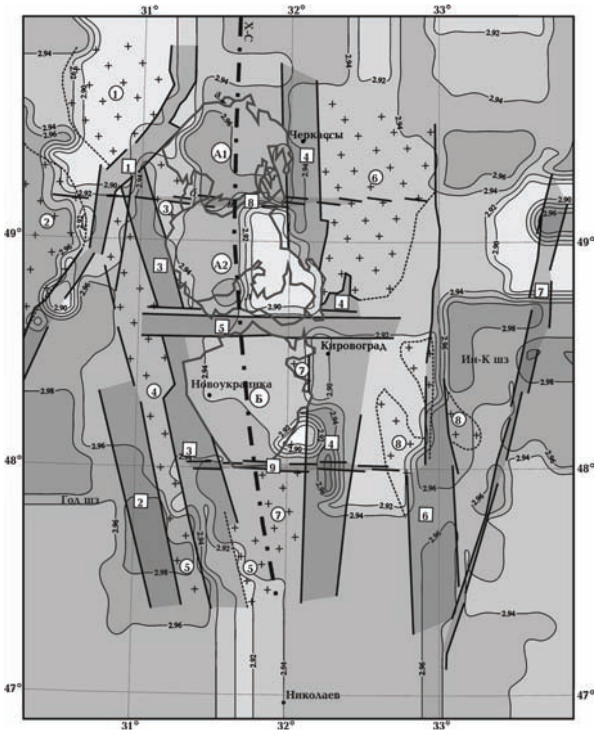
Рис. 7. Схема распределения плотности ( \text{г/см}^3 ) на глубине 30 км. Условные обозначения см. на рис. 1.
