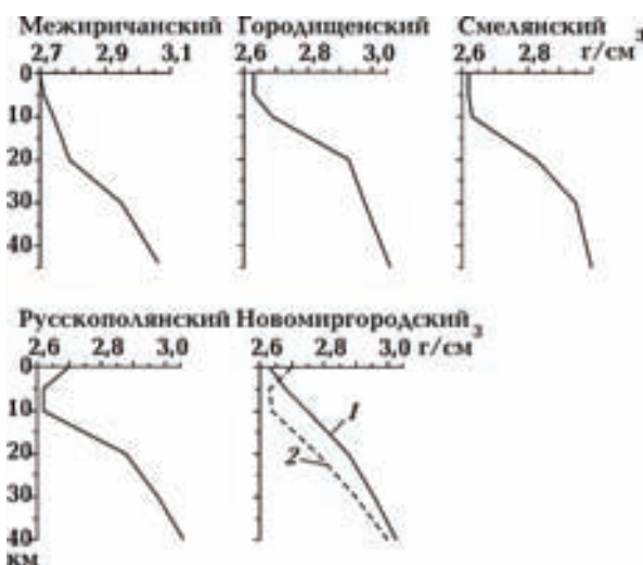
Рис. 10. Изменение плотности с глубиной в массивах габро-анортозитов. Расположение точек см. на рис. 1.
