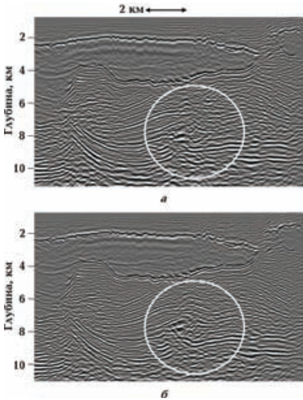
Рис. 3. Результаты миграции в обратном времени в Мексиканском заливе до (а) и после (б) уточнения скорости под солью с помощью сканирования временных задержек изображения.
