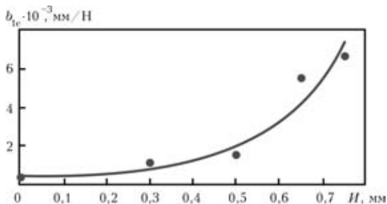
Рис. 5. Зависимость податливости шлицевого соединения b_{1c} от величины износа H
