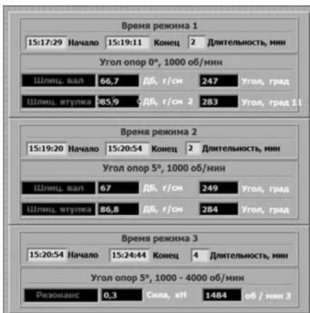
Рис. 2. Вид экрана ПК в режиме испытаний на этапе диагностики
