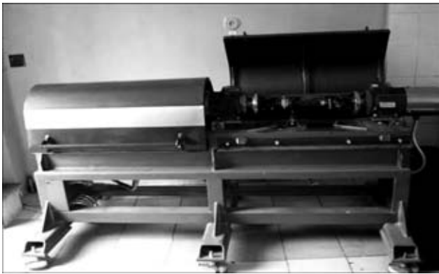
Рис. 1. Общий вид стенда «ВИК-4000»
