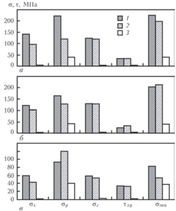
Рис. 10. Максимальные (по модулю) напряжения в материале 1 (а), 2 (б) и мягкой прослойки (в) узлов В-В при температурно-силовом (1), температурном (2) и силовом (3) нагружении с большим ТКЛР, т. е. сварка с термоциклированием под давлением в узлах с мягкой прослойкой обеспечивает более равномерное распределение пластических деформаций в прослойке.
