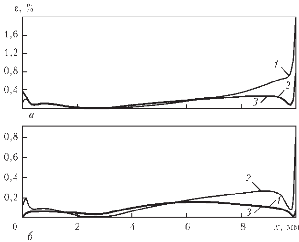
Рис. 9. Эпюры пластических деформаций в материале прослойки на стыке с соединяемыми материалами 1 (а) и 2 (б) в узлах В-В при температурно-силовом (1), температурном (2) и силовом (3) нагружении
