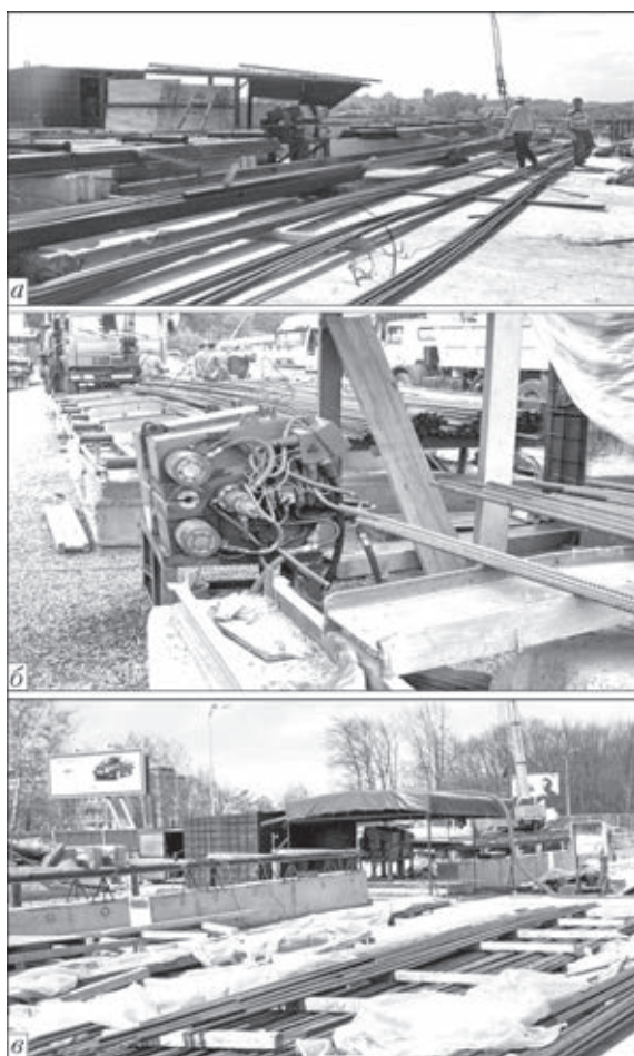
Рис. 7. Макеты линий для сварки арматуры на строительной площадке Подольского мостового перехода через р. Днепр (а), ригелей VIP-сектора НСК «Олимпийский» (б) и подъездной эстакады терминала D аэропорта «Борисполь» (в)
