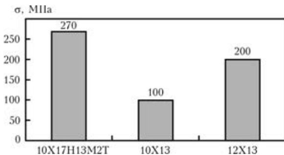
Рис. 3. Зависимость остаточных напряжений в околошовной зоне от материала плакирующего слоя
