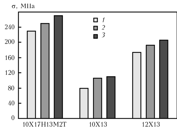
Рис. 4. Влияние толщины плакирующего слоя на остаточные напряжения в околошовной зоне: 1 — \delta = 5 мм; 2 — 7; 3 — 10
