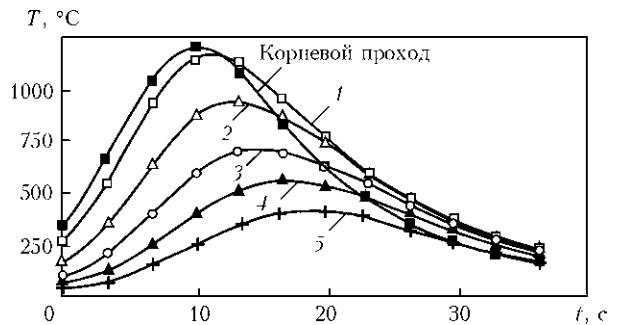
Рис. 4. Температурные циклы на внутренней поверхности при корневом проходе и последующих слоях (1–5)
