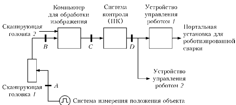
Рис. 5. Схема обработки данных для двух роботов (от сканирующей головки до сварочного робота)
