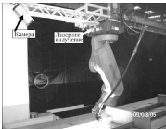
Рис. 7. Внешний вид робота с системой автоматизированного программирования путем обработки изображений, используемого для выполнения работ на судовой верфи
