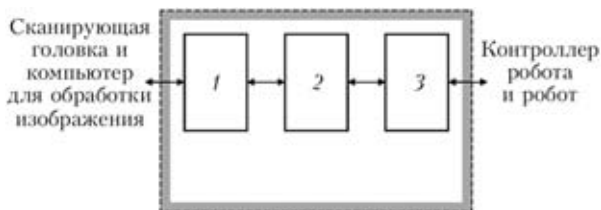
Рис. 4. Схема модулей управления системы обработки изображений при программировании робота: 1 — математическое обеспечение для обработки изображений; 2 — система программирования в неавтономном режиме; 3 — макроуправление сервером управления
