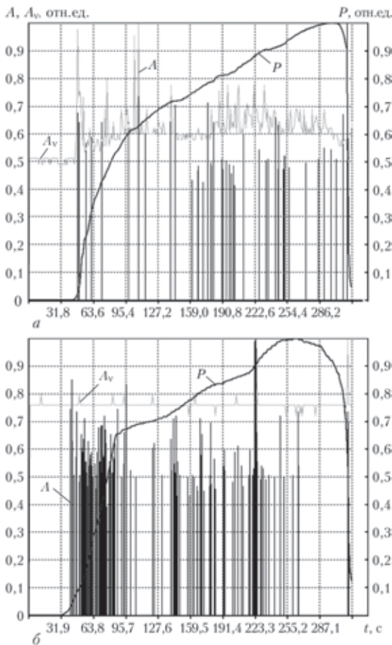
Рис. 18. Сопоставление сигналы акустической эмиссии в растягиваемых образцах из стали 15Х1М1Ф при комнатной температуре (а) и 500 °С (б) (А — амплитуда; Av — амплитуда непрерывной эмиссии; P — нагрузка)
