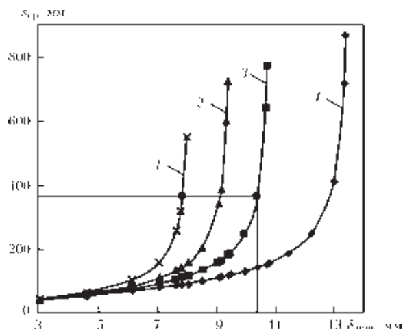
Рис. 17. Зависимость критической длины дефекта типа локального утонения s_{кр} от минимальной допустимой толщины \delta_{мин} стенки трубы 1420 \times 20 мм из стали 17Г1С при различном внутреннем давлении: 1 — 4,5; 2 — 5,25; 3 — 6,0; 4 — 7,5 МПа
