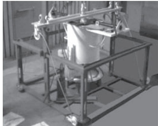
Рис. 20. Модуль для соединения разрушенных труб скважин модуля с места закрепления благодаря имеющимся в конструкции модуля необходимым отверстиям, которые обеспечивают свободное вытекание интенсивного потока нефти в окружающую среду. Затем эти отверстия модуля перекрываются. Для этого используются гидроцилиндры и специальные шторы, предусмотренные конструкцией модуля. После завершения работы гидроцилиндров и перекрытия отверстий модуля нефть направляется в нужном направлении по трубопроводу. Таковы разработки института, предназначенные для современной энергетики. Исследования и создание новых технологий продолжают.
