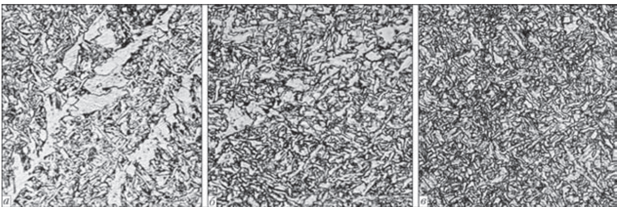
Рис. 13. Микроструктура ( \times 500 ) металла швов труб из стали класса прочности К60, выполненных с применением различных сварочных материалов: а – Mn–Mo система легирования, кислый плавный флюс, полигонального феррита 20...25 %; игольчатого 35...45 %; KV_{-30} = 27...30 Дж/см 2 ; б – Mn–Ni–Mo система легирования, алюминатный агломерированный флюс небольшой основности, полигонального феррита 3...5 %, игольчатого 75...80 %; KV_{-30} = 80...100 Дж/см 2 ; в – Mn–Mo–Ti–V система легирования, алюминатный агломерированный флюс небольшой основности, полигонального феррита менее 1 %, игольчатого 85...90 %; KV_{-30} = 180...200 Дж/см 2
