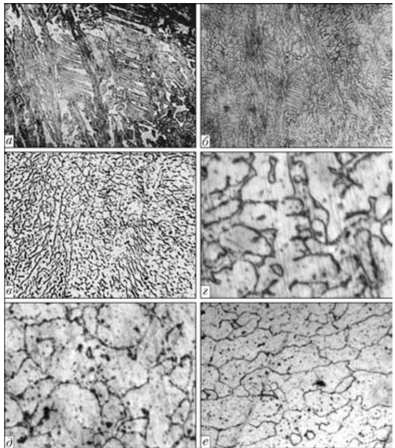
Микроструктуры ( \times 550 ) хромомарганцевого наплавленного металла с различным содержанием марганца: а — Св-12Х13 (эталон); б — 2 % Мп; в — 4; д — 8; е — 12
