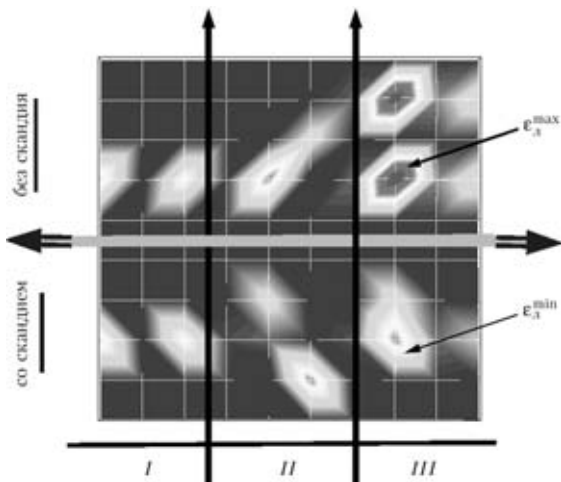
Рис. 6. Диаграммы распределения зон локализации деформации \epsilon_{л} в металле шва сплава 1460 с использованием присадочной проволоки Св1201 и Св1201+Sc после сварки (I) и термообработок при T = 150\text{ }^{\circ}\text{C} , t = 22\text{ ч} (II) и T = 350\text{ }^{\circ}\text{C} , t = 1\text{ ч} (III)
