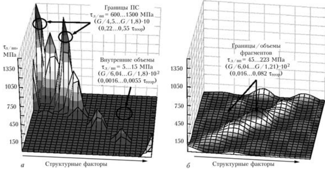
Рис. 8. Распределение локальных внутренних напряжений \tau_{л/вн} в металле шва типа Св1201 (а), Св1201+0,5%Sc (б) (термообработка при T = 350 °С, t = 1 ч) после внешнего динамического нагружения
