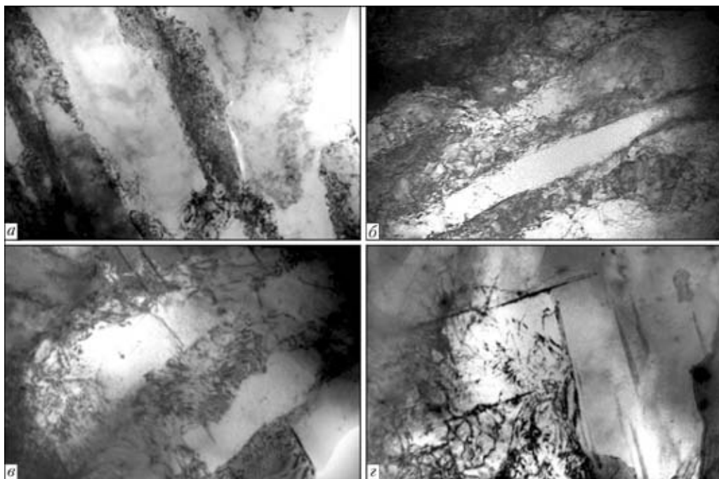
Рис. 7. Изменение тонкой структуры термообработанного ( T = 350\text{ }^{\circ}\text{C} , t = 1\text{ ч} ) металла шва сплава 1460 в условиях динамического нагружения в зависимости от способа легирования (без скандия и с ним): а, б — мощные ПС в металле без скандия (соответственно \times 20000 и \times 30000 ); в, г — фрагментация структуры вследствие блокирования ПС фазами скандия в металле со скандием, \times 30000
