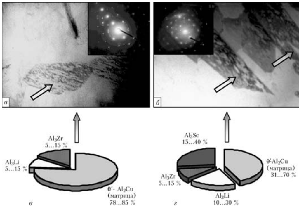
Рис. 9. Изменение (в условиях термообработки при T = 350 °С, t = 1 ч) структуры (а, б — \times 50000 ) и состава (в, з) \theta' -фазовых образований в металле шва сварного соединения сплава 1460 в зависимости от способа легирования без скандия (а, в) и с ним (б, з)
