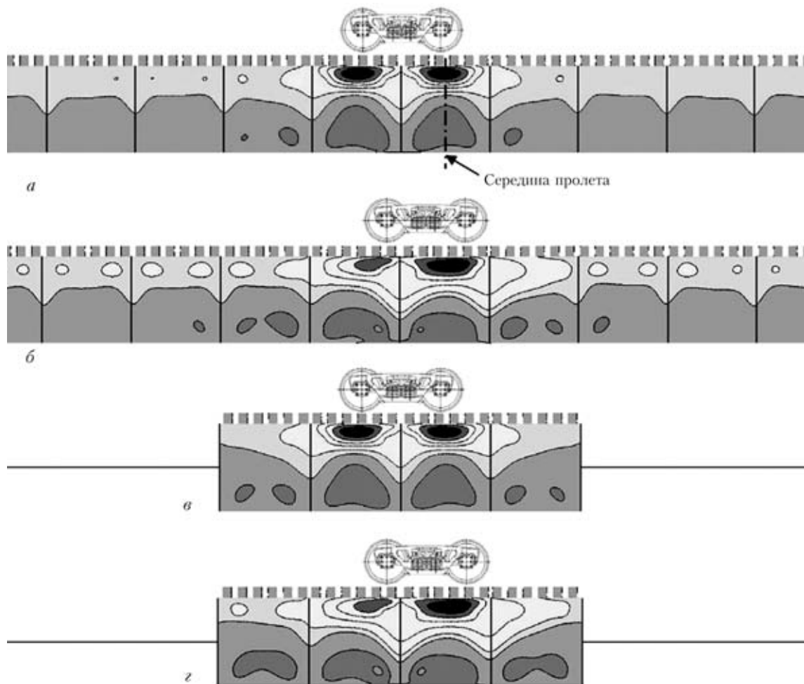
Рис. 8. Изополя поперечных перемещений вертикальной стенки в отсеках по первой ( а, б ) и второй (предлагаемой) модели ( в, г )
