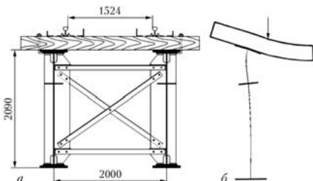
Рис. 5. Поперечное сечение сварного пролетного строения моста (а) и деформация его стенки из плоскости (б)
