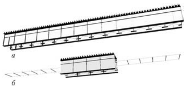
Рис. 7. Расчетные модели цельносварного пролетного строения (пояснения в тексте)
