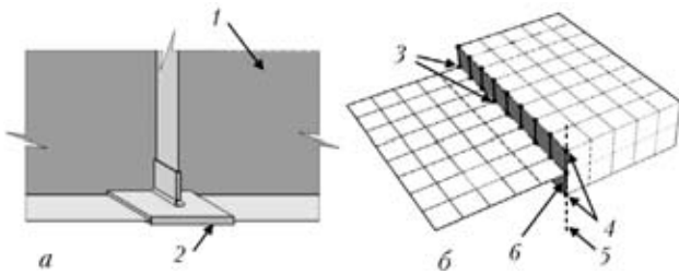
Рис. 4. Замена оболочечных КЭ трехмерной моделью (а) и введение АЖТ между оболочечными и трехмерными КЭ (б): 1 — оболочечная модель фрагмента конструкции; 2 — трехмерная модель узла; 3 — ведущие узлы; 4 — ведомые узлы; 5 — грань с ведущим и ведомыми им узлами; 6 — АЖТ
