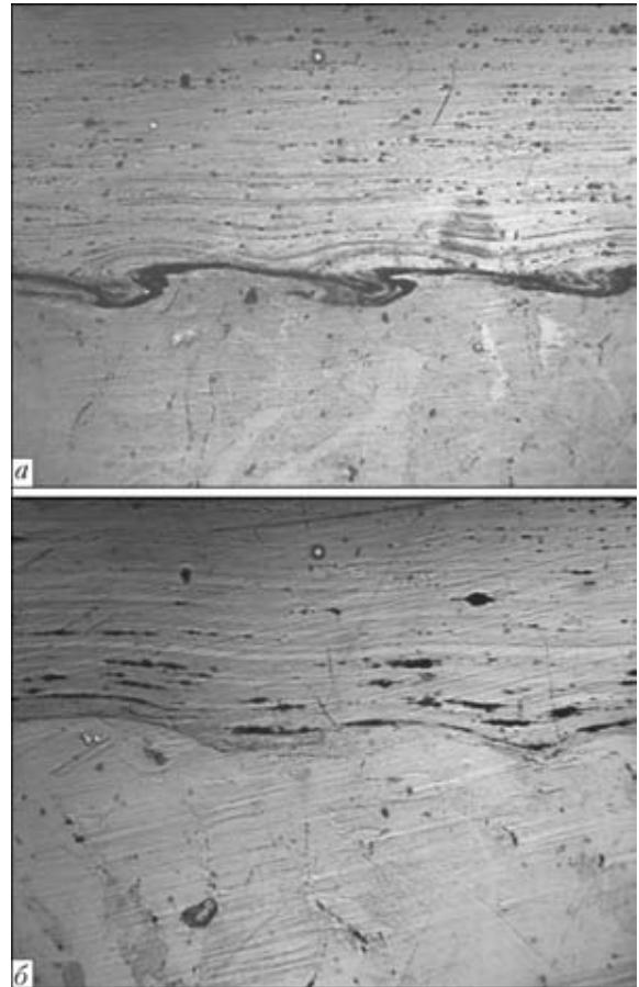
Рис. 4. Типичная микроструктура (×100) соединения сплава 7018 без термообработки лакирующей пластины (а) и аналога сплава 7050 с применением новой технологии сварки взрывом (б)
