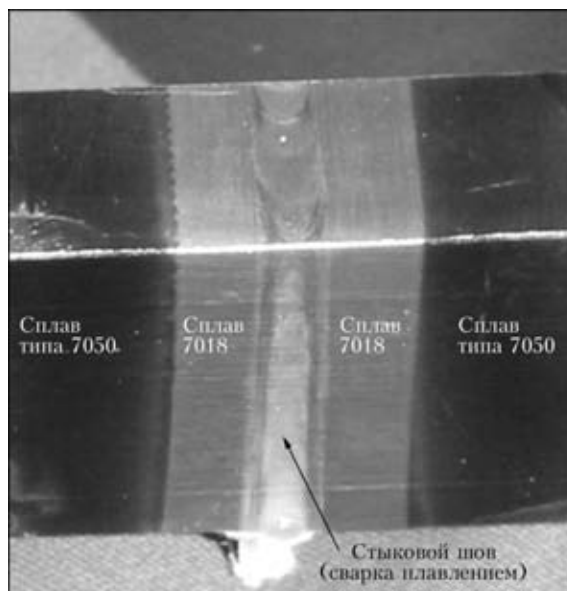
Рис. 5. Макроструктура стыкового комбинированного соединения высокопрочного трудносвариваемого алюминиевого сплава
