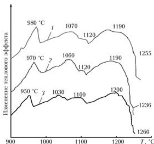
Рис. 4. Кривые ДТА, полученные при кристаллизации расплавленных слитков комплексных припоев № 1 + NiC 2 + 60 % Rene-142 с различным содержанием кремнийсодержащей составляющей NiC 2 : 1 — припой № 13; 2 — № 14; 3 — № 12
