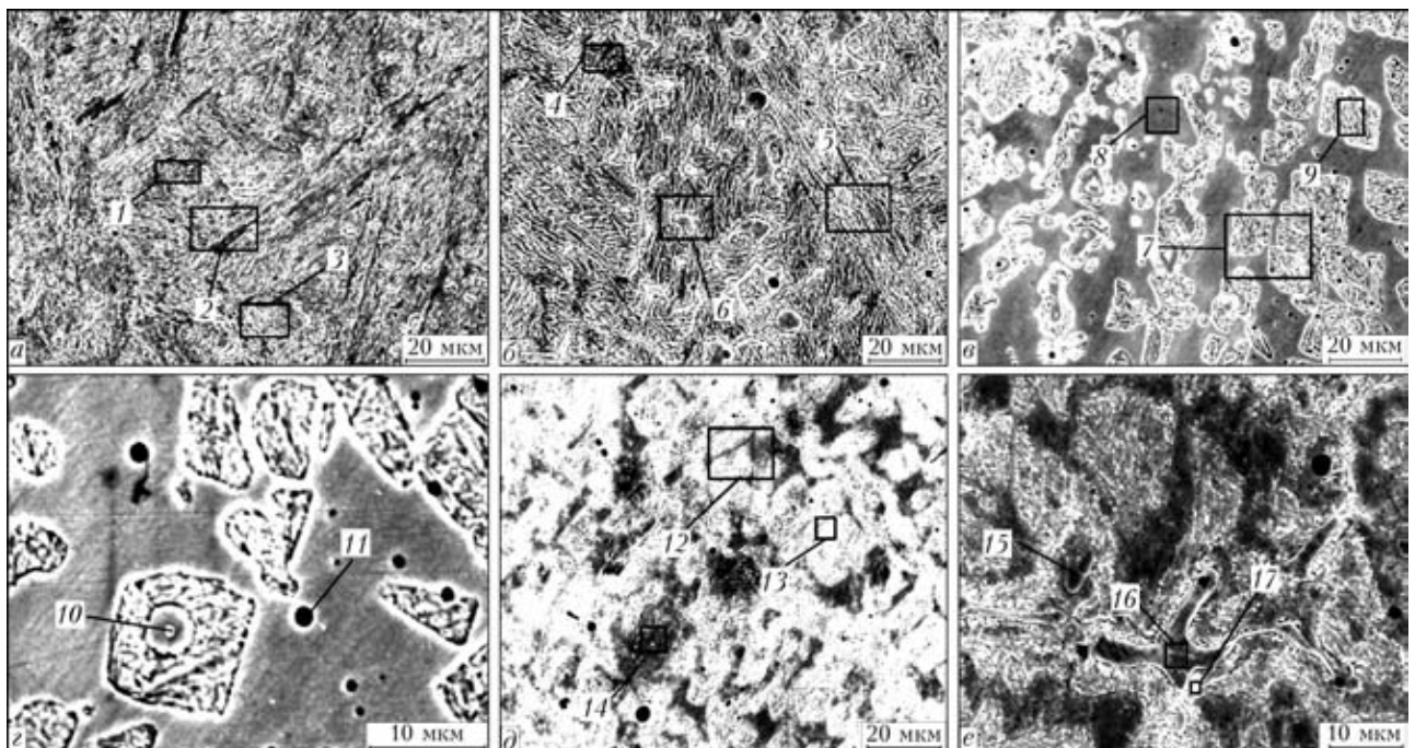
Рис. 5. Микроструктура образцов наплавленного металла 30Х2М2НСГФ без фосфора (а) и с 0,57 (б), 0,89 (в, д), 1,42 мас. % (е) Р (см. табл. 3)
