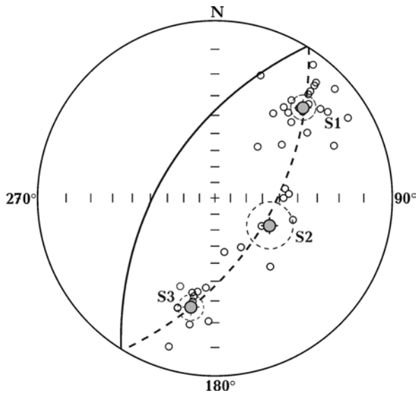
Рис. 5. Стереографическая проекция направлений компонент S1, S2, S3 для пород Коновской свиты верхнего силура. Приведено положение большого круга перемagnetизования относительно полученных направлений.
