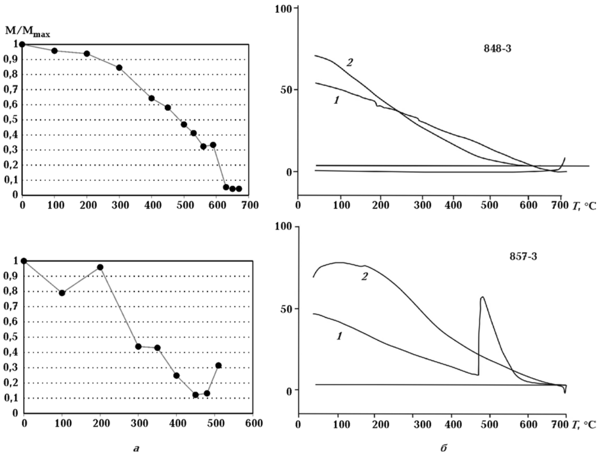
Рис. 6. Примеры разрушения: нормированной ЕОН в процессе ступенчатого терморазмагничивания (а); остаточной намагненности насыщения в процессе непрерывного нагрева (1 — первый нагрев, 2 — второй нагрев) образцов коновской свиты верхнего силура (б).
