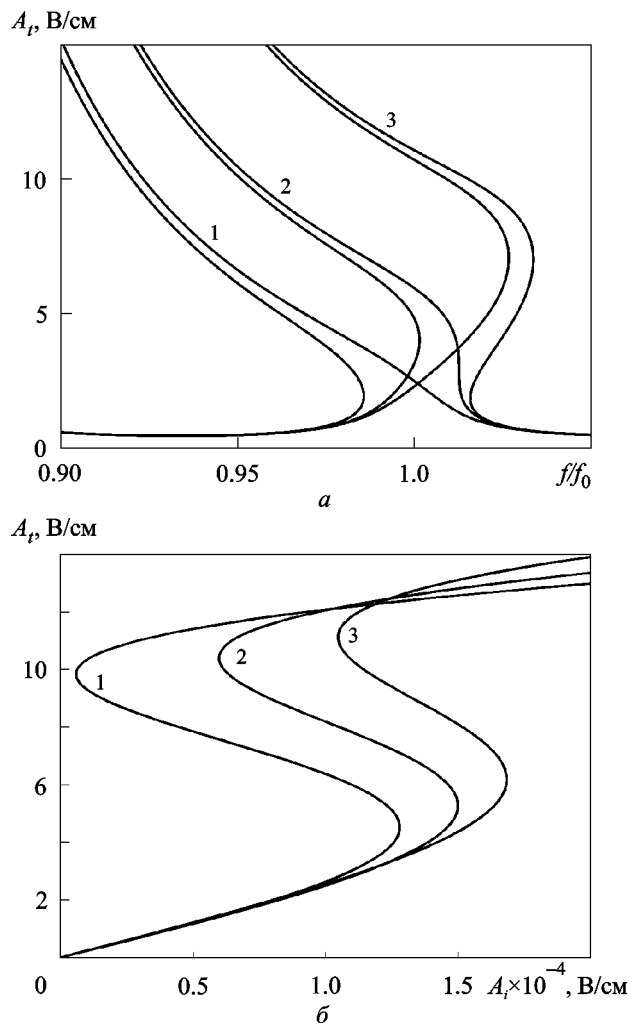
Рис. 4. Явление гистерезиса в брэгговском резонаторе с составным нелинейным слоем: а – зависимость амплитуды прошедшей волны от частоты при амплитуде падающей волны A_i = 2 \cdot 10^3 В/см для различных соотношений толщин подслоев с нелинейной диэлектрической проницаемостью, изменяющейся по возрастающему и убывающему законам (линия 1 – электрическая толщина первой части слоя h_{n1} = 0.5h , линия 2 – h_{n1} = 0.4h , линия 3 – h_{n1} = 0.25h ); б – зависимость амплитуды прошедшей волны от амплитуды падающей волны при различных значениях частот (линия 1 – f/f_0 = 1.07 , линия 2 – f/f_0 = 1.08 , линия 3 – f/f_0 = 1.09 )
