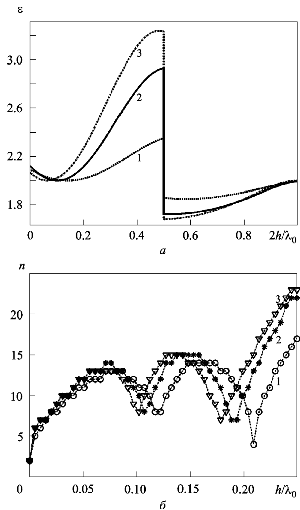
Рис. 5. Расчет диэлектрической проницаемости нелинейного составного резонансного слоя: а – распределение диэлектрической проницаемости при различных значениях частоты падающей электромагнитной волны (линия 1 – f/f_0 = 1.1 , линия 2 – f/f_0 = 1.05 , линия 3 – f/f_0 = 1.0 ); б – зависимость количества итераций от толщины слоя при различных значениях амплитуды падающей волны (линия 1 – A_i = 10^3 \text{ В/см} , линия 2 – A_i = 1.5 \cdot 10^3 \text{ В/см} , линия 3 – A_i = 2 \cdot 10^3 \text{ В/см} )
