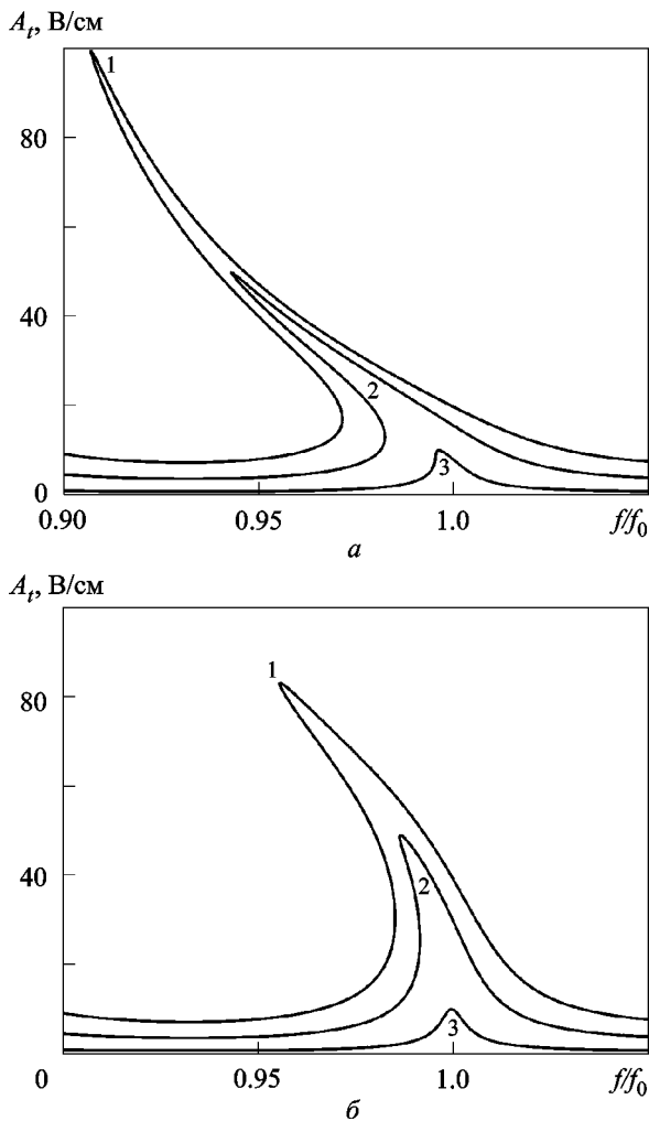
Рис. 6. Зависимость амплитуды прошедшей волны от частоты для брэгговского резонатора при различных амплитудах падающей волны: a – положение сосредоточенного элемента симметрично (линия 1 – A_i = 100 В/см, линия 2 – A_i = 50 В/см, линия 3 – A_i = 10 В/см); б – точка включения сосредоточенного элемента делит центральный резонансный слой на подслои с электрическими толщинами \lambda_0/10 и 4\lambda_0/10 (линия 1 – A_i = 100 В/см, линия 2 – A_i = 50 В/см, линия 3 – A_i = 10 В/см)
