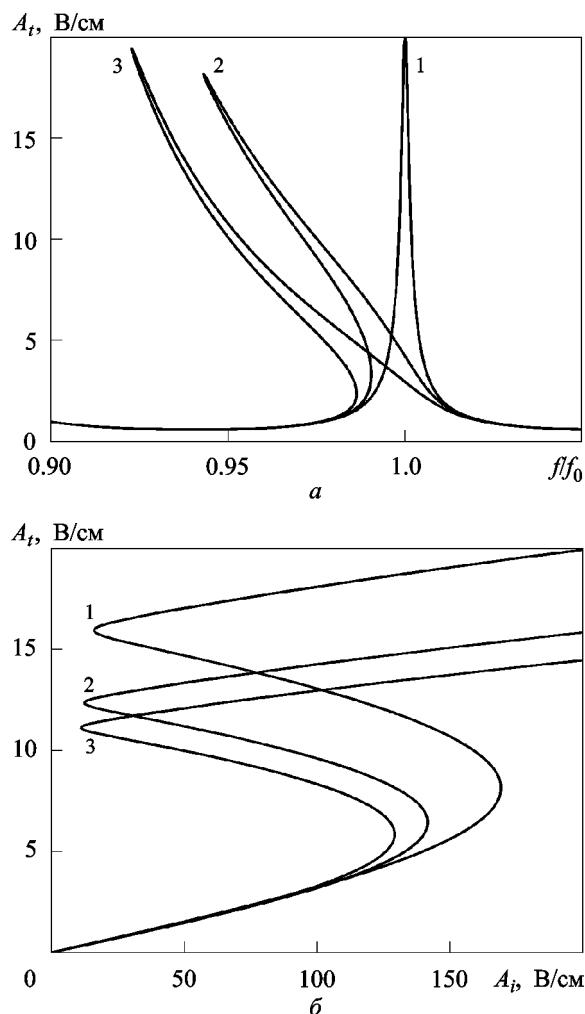
Рис. 2. Явление гистерезиса в брэгговском резонаторе с нелинейным слоем: а – зависимость амплитуды прошедшей волны от частоты при амплитуде падающей волны A_i = 20 В/см для различных соотношений толщин линейной и нелинейной частей резонансного слоя (линия 1 – линейный случай, линия 2 – электрическая толщина нелинейного слоя h_1 = 0.45h , электрическая толщина линейного слоя h_2 = 0.55h , линия 3 – электрическая толщина нелинейного слоя h_1 = 0.95h , электрическая толщина линейного слоя h_2 = 0.05h ); б – зависимость амплитуды прошедшей волны от амплитуды падающей волны при различных значениях частот (линия 1 – f/f_0 = 1.09 , линия 2 – f/f_0 = 1.08 , линия 3 – f/f_0 = 1.07 )
