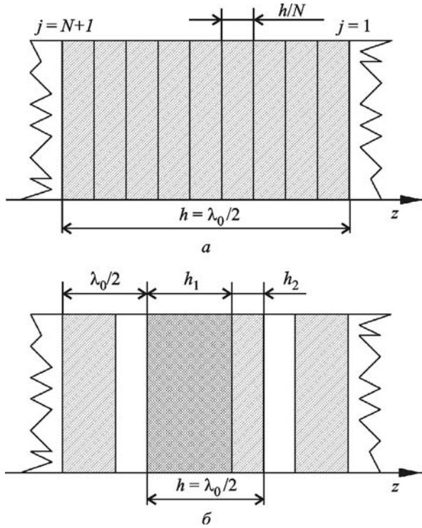
Рис. 1. Конструкция слоистого брэгговского резонатора: a – разбиение центрального резонансного нелинейного слоя с оптической толщиной h = \lambda_0/2 на N подслоев (направление стратификации совпадает с осью z ); б – конструкция брэгговского резонатора с резонансным слоем, состоящим из двух слоев с электрическими толщинами h_1 и h_2 и различными диэлектрическими проницаемостями (электрическая толщина периода h = \lambda_0/2 )
