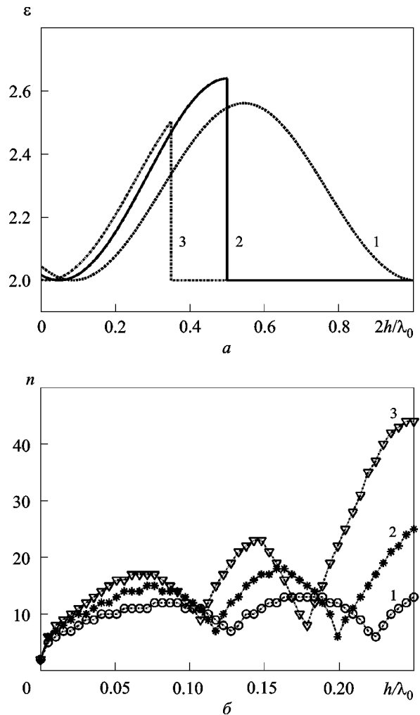
Рис. 3. Расчет диэлектрической проницаемости слоя с керровской нелинейностью: а – распределение диэлектрической проницаемости составного нелинейного слоя при различных соотношениях электрических толщин линейного и нелинейного слоев (линия 1 – h_1 = h , линия 2 – h_1 = 0.5h , линия 3 – h_1 = 0.35h ); б – зависимость количества итераций от толщины нелинейного слоя при различных значениях амплитуды падающей волны (линия 1 – A_i = 10^3 В/см, линия 2 – A_i = 1.5 \cdot 10^3 В/см, линия 3 – A_i = 2 \cdot 10^3 В/см)
