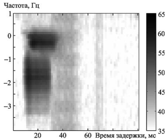
Рис. 3. Усредненная спектрограмма сигнала РВМ, полученная для периода 19:20–19:30 местного времени 22.09.2010 г. на частоте 9996 кГц
