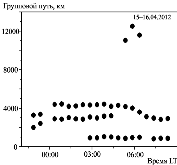
Рис. 9. Длина группового пути различных мод импульсного сигнала на частоте 9996 кГц на трассе антенны РВМ – РАО 15–16.04.2012 г.
