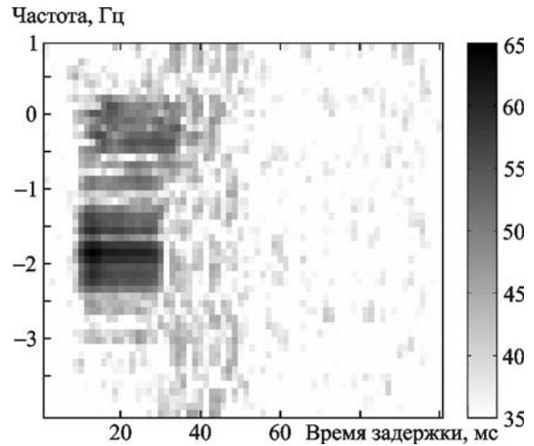
Рис. 2. Спектрограмма сигнала РВМ, полученная в интервале 19:23:00–19:23:10 местного времени 22.09.2010 г. на частоте 9996 кГц
